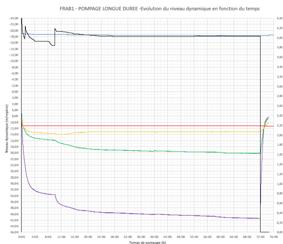
Figure 2 : Acquisitions d'un essai de pompage
