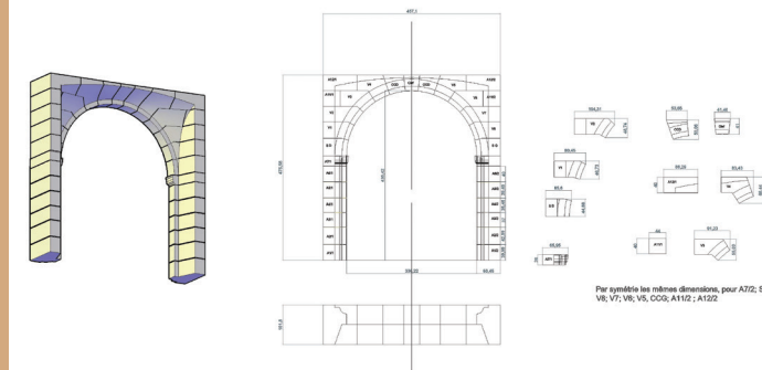
Arrière Voussure de Marseille Dimensions pour blocs capables En cm Projet EASMS pour Marmoutier 2019
